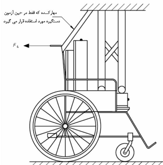
الف- تجهیزات کلی بارگذاری
