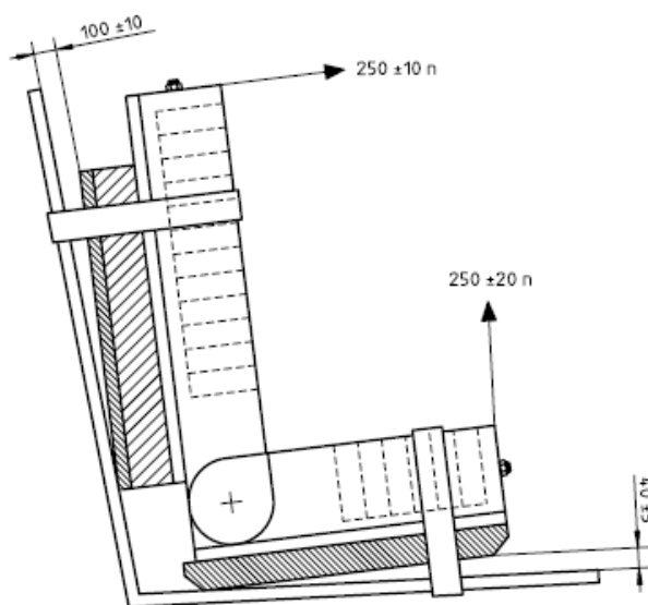
شکل ۲۰-ب - کشش قبلی مهارکننده ها برای آزمون خستگی توسط آدامک آزمون ۷۵ کیلوگرمی
