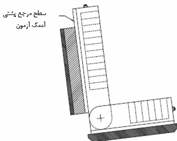
شکل ۴- سطح مرجع پستی آدمک آزمون
