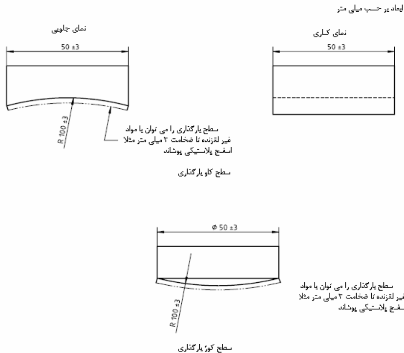
شکل ۱- سکوه های بارگذاری برای بارهای ساکن
