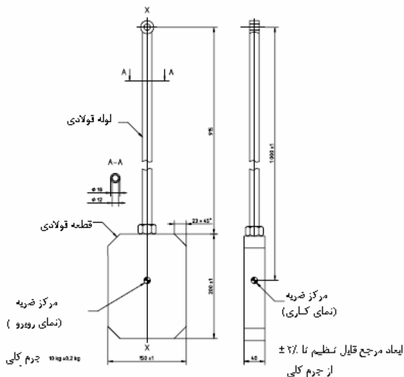
شکل ۳- پاندول آزمون ضربه به طوقه دستی
