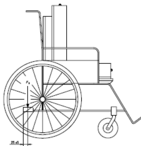
شکل ۹- بار وارده به اهرم های کج کننده
