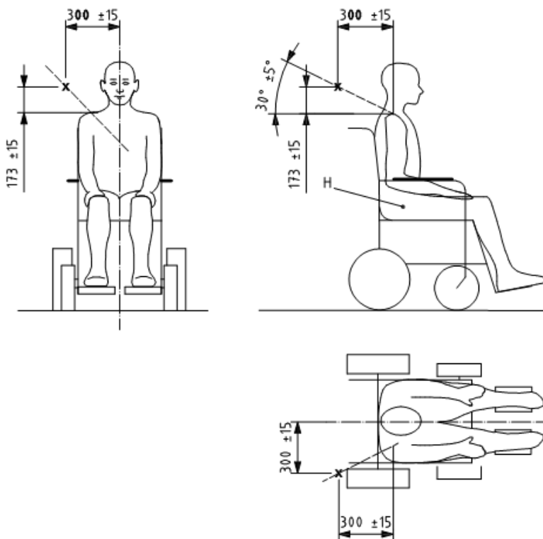
شکل ۱- موقعیت آزمون نقطه تکیه‌گاه بالایی کمر بند محافظ شانه‌ای یا نقطه راهنما و زوایای کمر بند محافظ شانه‌ای
